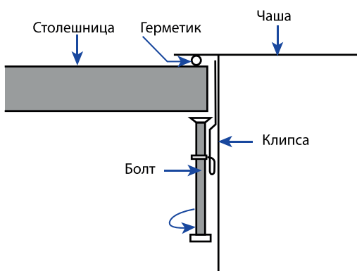
Врезной монтаж
