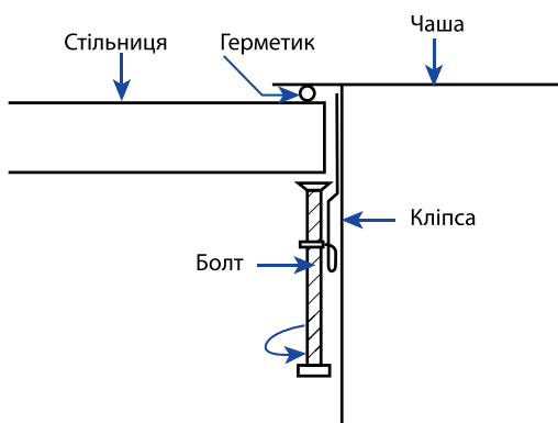
Врізний монтаж
